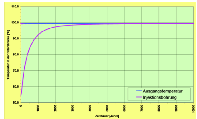
Abb. 9: Wärmeregeneration in der Filterstrecke der Injektionsbohrung TH1 über einen Zeitraum von 10.000 Jahren.
