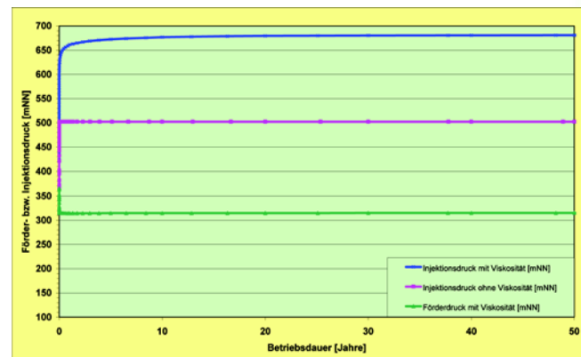
Abb. 6: Zeitliche Entwicklung des Grundwasserpotenzials in Förder- und Injektionsbohrung
